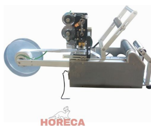
Этикетировщик HL-50 с датером Hualian Machinery
