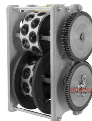
Формующий модуль в сборе пельменного аппарата JGL-160, Имитация ручной лепки, 10 гр Foodatlas
