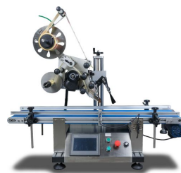
Автоматический этикетировщик для плоских поверхностей HLKBL-150 Hualian Machinery
